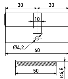
Цилиндр
