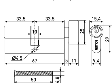
Цилиндр
