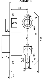
Замок
