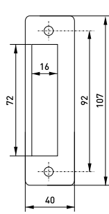
Ответная планка
