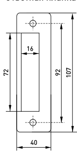
Ответная планка
