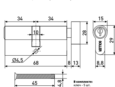
Цилиндр с заверткой
