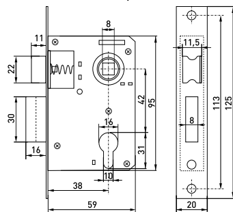
Замок врезной
