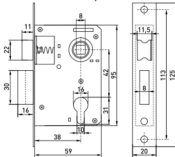
Замок врезной
