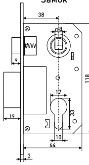
Замок
