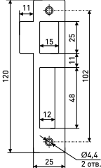
Ответная планка
