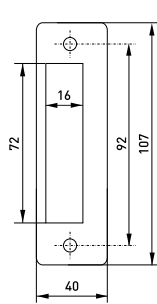
Ответная планка
