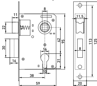
Замок врезной
