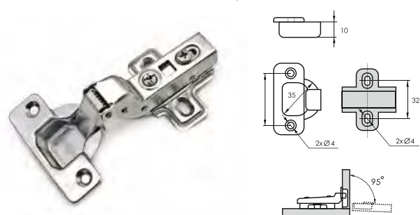
1111 Петля вкладная с доводчиком clip-on
