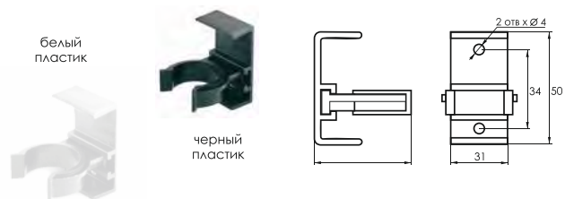
Клипса+подклипник для опоры
