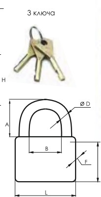
BC-203 Замок навесной с кодированием BC-304 BC-404
