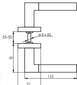
ZF11-R280 Комплект дверных ручек SOLLER ЦАМ/алюминий
