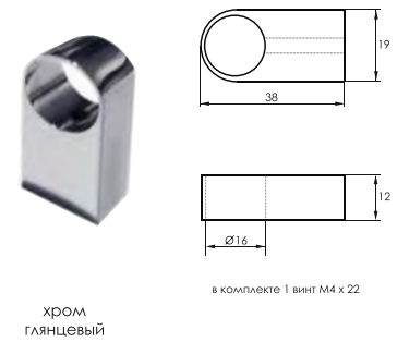
1274 Держатель рейлинга сквозной d-16
