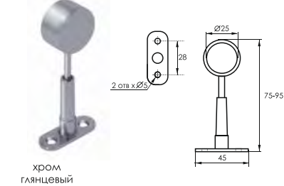
R-50AR Держатель дистанционный регулируемый торцевой d-25
