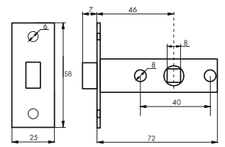
в комплекте: 4 шурупа 3,9 x 18 1 ответная планка
