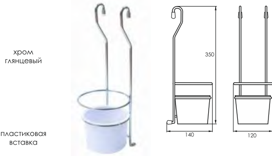
KS-2032 Кружка на рейлинг
