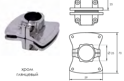
302T Муфта с 3-мя направлениями T-образная d-25
