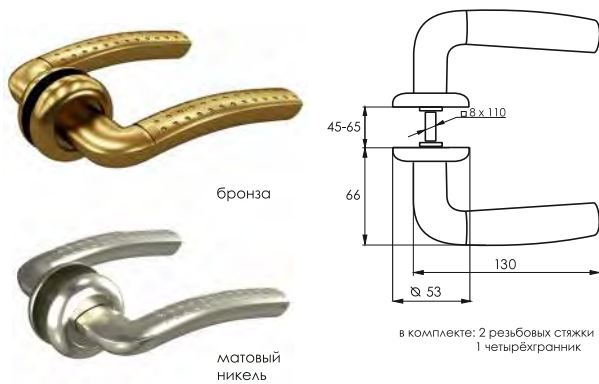
ZY-503 Комплект дверных ручек SOLLER ЦАМ/алюминий
