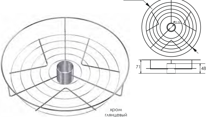
Полка центральная (350x63)
