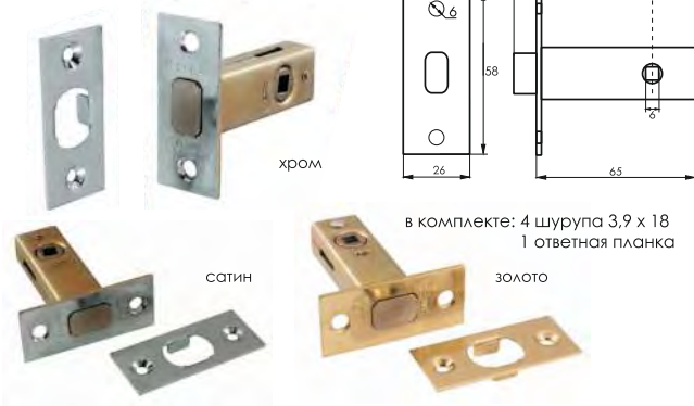
002 BK-HD Задвижка дверная
