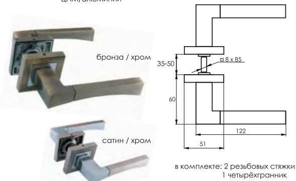
ZF11-R280 Комплект дверных ручек SOLLER ЦАМ/алюминий
