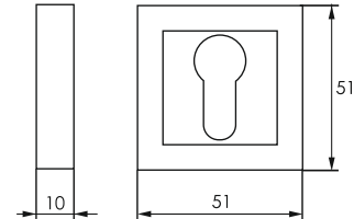
в комплекте 8 винтов M4x22
