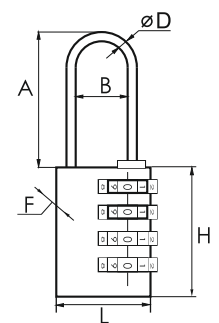
BC-203 Замок навесной с кодированием BC-304 BC-404
