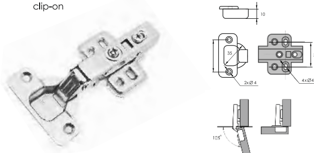
1112 Петля накладная с длинным доводчиком clip-on
