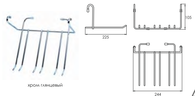
KS-2022 Полка для бокалов
