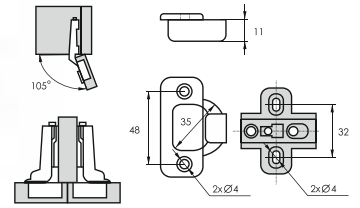
362 AB Петля мебельная полунакладная slide-on
